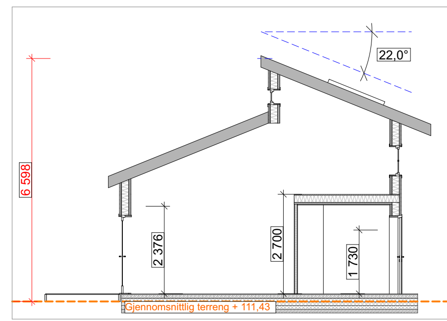
Snitt 2 leil 05
