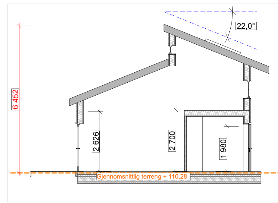
Snitt 2 leil 03
