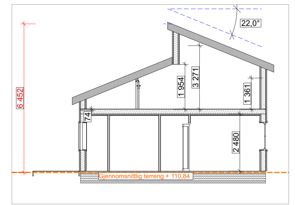
Snitt 1 leil 03
