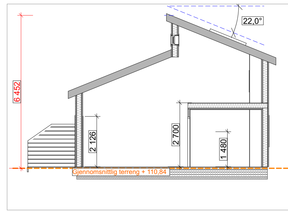
Snitt 2 leil 01
