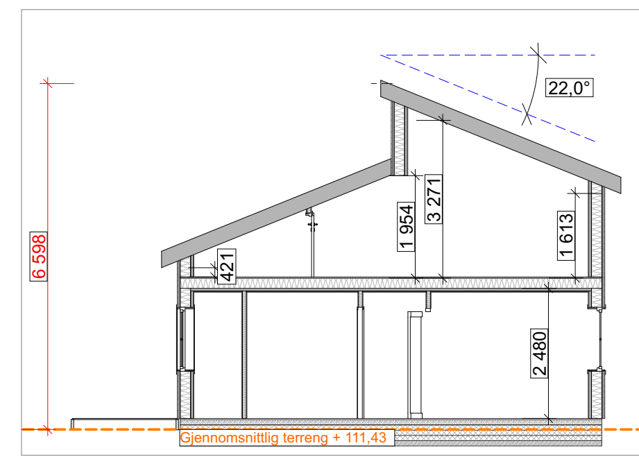
Snitt 1 leil 07
