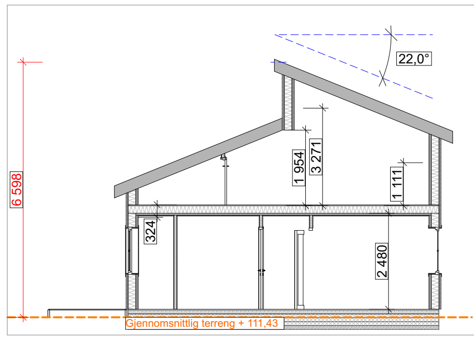
Snitt 1 leil 05
