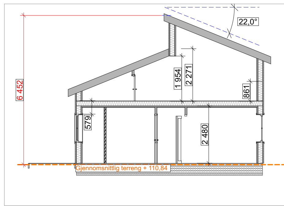
Snitt 1 leil 01
